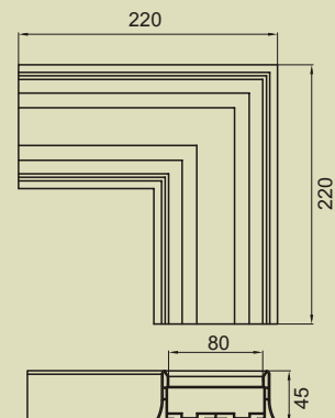
σύνδεσμος στρωτήρα για 80 mm connection corner for 80 mm
