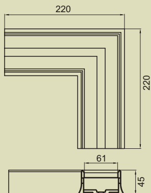
σύνδεσμος στρωτήρα για 60 mm connection corner for 60 mm
