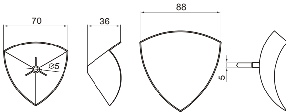
εσωτερική γωνία υγειονομικής internal corner cap
