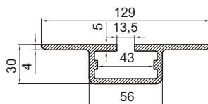
πολυεστερικό προφίλ "ΩΜΕΓΑ" polyester "OMEGA" profile
