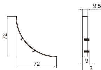
τελείωμα υγειονομικής γωνίας end cap
